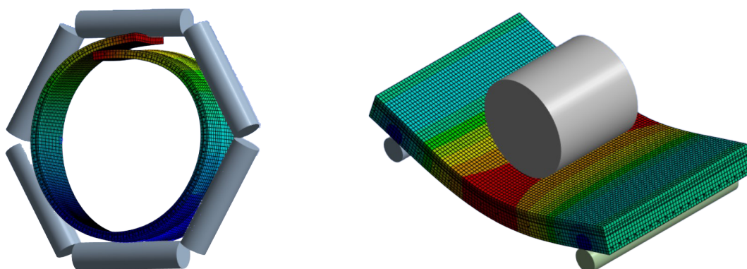
Exemplo de modelagem de uma correia tubular 3D usando nosso software
