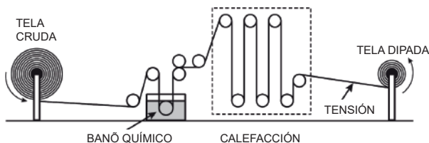
Figura 1: Ilustración esquemática del proceso de Dipping
