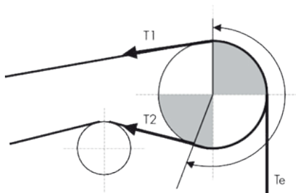
Figura 8: Tensiones en el tambor de accionamiento
